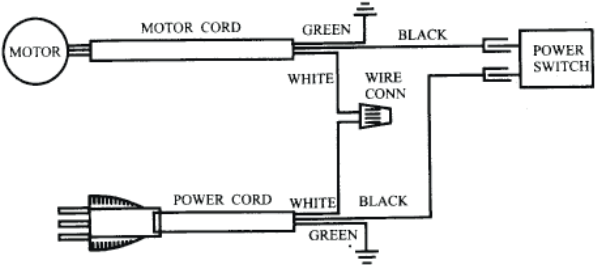
Diγράμα para el TB658B / TB658B Speed Chart
