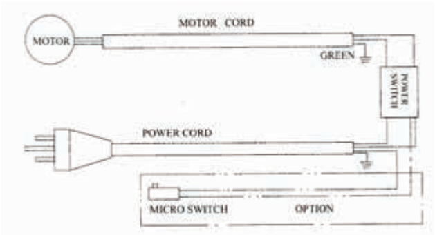
Diγράμα para el TC658B / TC658B Speed Chart
