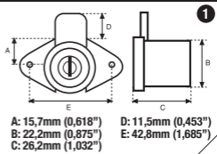
Dimensiones de la Cerradura Lock Dimensions
