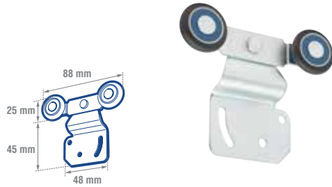
Doble riel superior.
